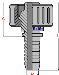
23.6213 Fêmea Métrica em Latão c/ Anel Plástico para Lavadoras (tipo Kaercher)
